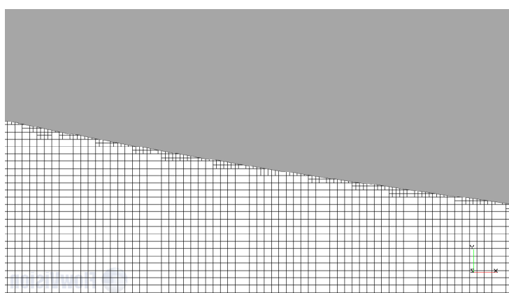
Рис. 11. Внешний вид сечения расчетной сетки при адаптации к решению с использованием градиента скорости а) для ЦАГИ Р-30А-15, б) для NASA 0012.
