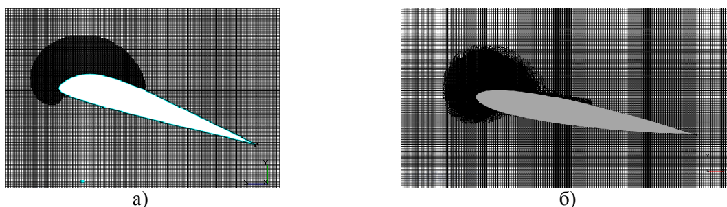
Рис. 10. Внешний вид сечения расчетной сетки при проведении адаптации к решению с использованием градиента давления а) для ЦАГИ Р-31А-15, б) для NASA 0012.
