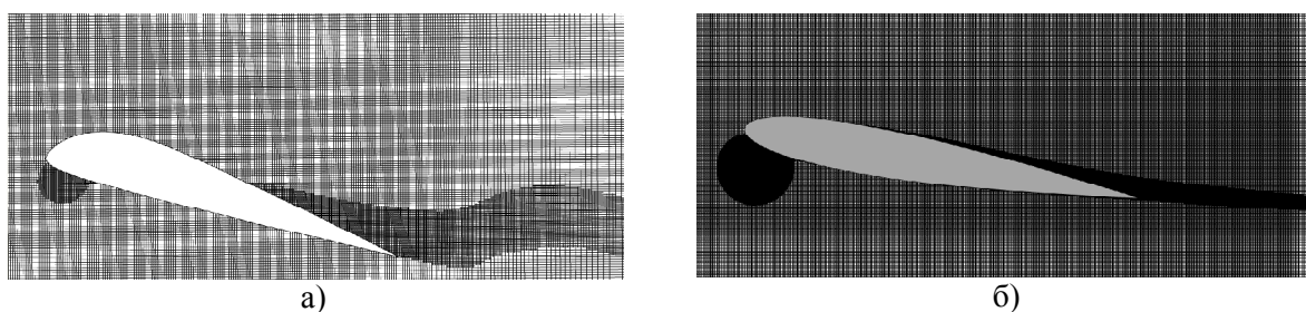
Рис. 13. Сечение расчетной сетки при адаптации по значению скорости а) для ЦАГИ Р-30А-15, б) для NASA 0012.
