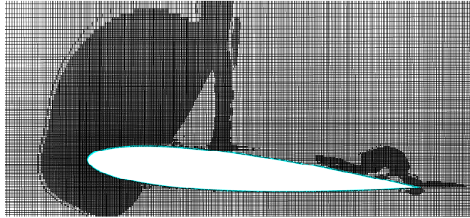
Рис. 16. Внешний вид сечения расчетной сетки при проведении адаптации к решению с использованием градиента скорости для NACA 0012 при трансзвуковом режиме обтекания.
