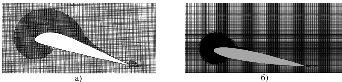
Рис. 11. Внешний вид сечения расчетной сетки при адаптации к решению с использованием градиента скорости а) для ЦАГИ Р-30А-15, б) для NASA 0012.
