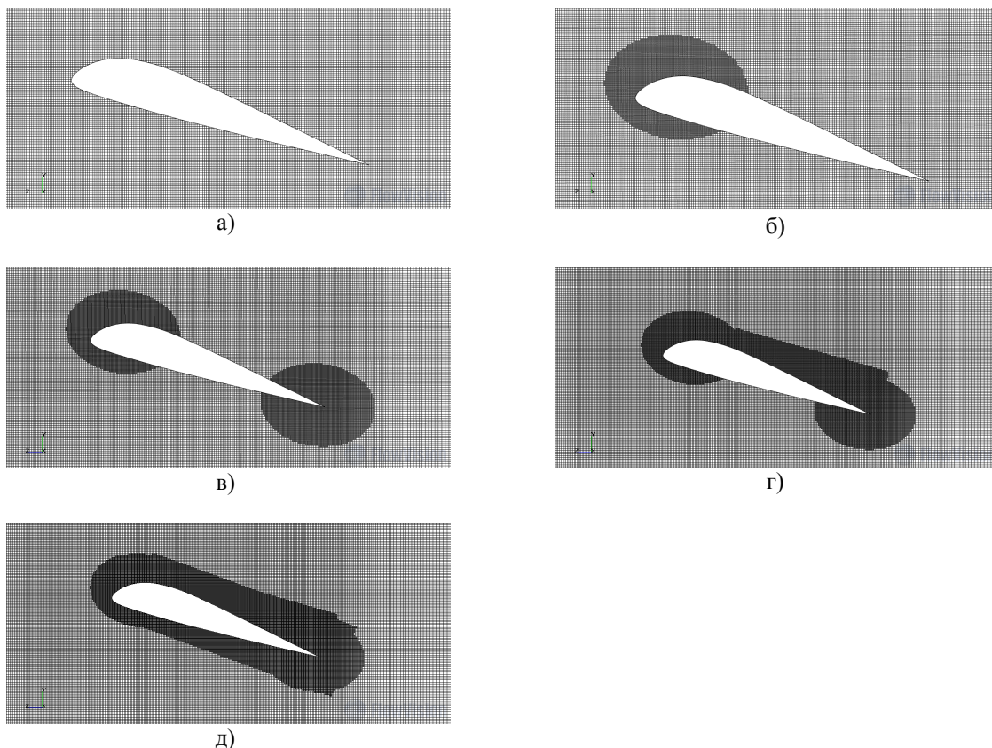
Рис. 6. Расчетные сетки при исследовании влияния адаптации различных областей около крылового профиля ЦАГИ Р-IIIА-15 на результаты решения: без адаптации (а), адаптация по передней кромке (б), адаптация по передней и задней кромке (в), адаптация по передней кромке, задней кромке и зоне отрыва потока (г), адаптация вокруг всего профиля (д).
