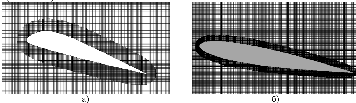
Рис. 14. Сечение расчетной сетки при адаптации по значению расстояния от стенки а) для ЦАГИ Р-IIIА-15 , б) для NASA 0012.
