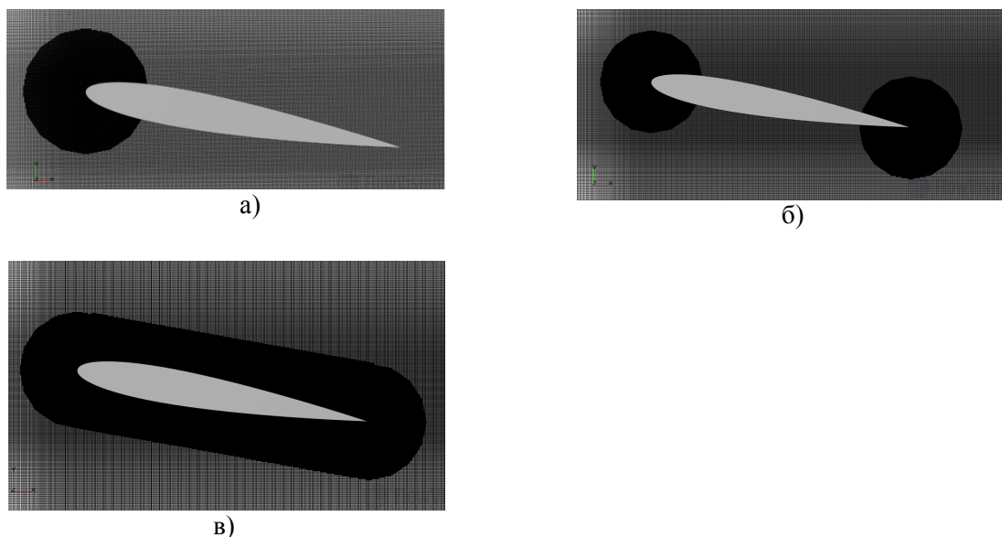
Рис. 5. Расчетные сетки для исследования влияния адаптации различных областей около крылового профиля NASA 0012 на результаты решения: с адаптацией рядом с передней кромкой профиля (а), с адаптацией рядом с передней и задней кромками (б), с адаптацией вокруг всего крылового профиля (в).
